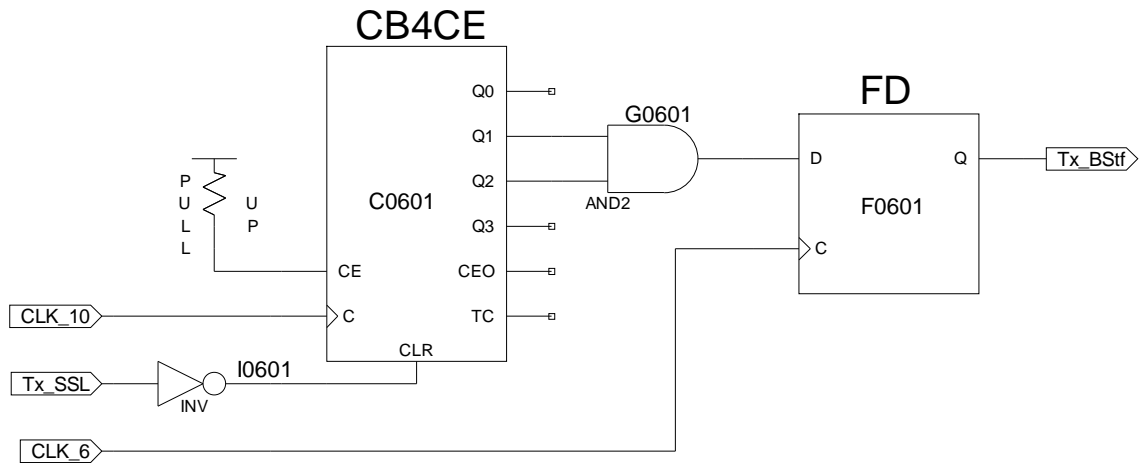
Rysunek 26: Schemat ideowy bloku wstawiania Bit Stuffing'u
