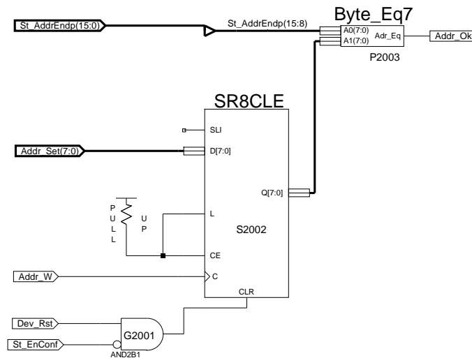
Rysunek 39: Schemat ideowy bloku sprawdzania zgodności adresu interfejsu ( St_Adr ).
