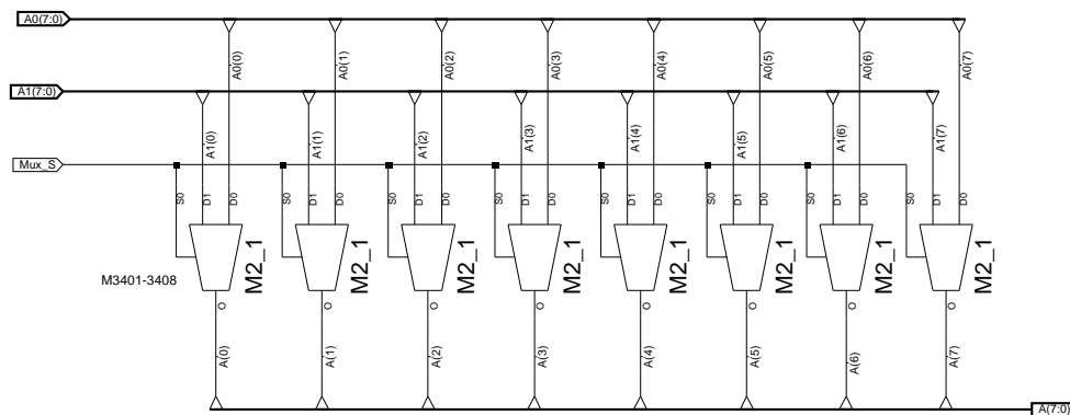
Rysunek 42: Multiplekser jednobajtowy - schemat ideowy ( Byte_Mux ).
