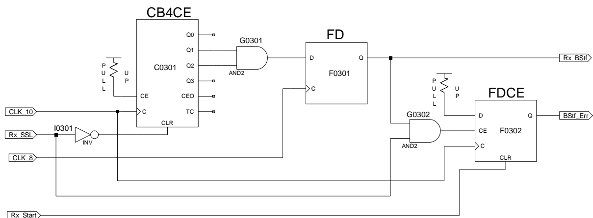
Rysunek 18: Schemat ideowy bloku wycinania bitów synchronizacyjnych
