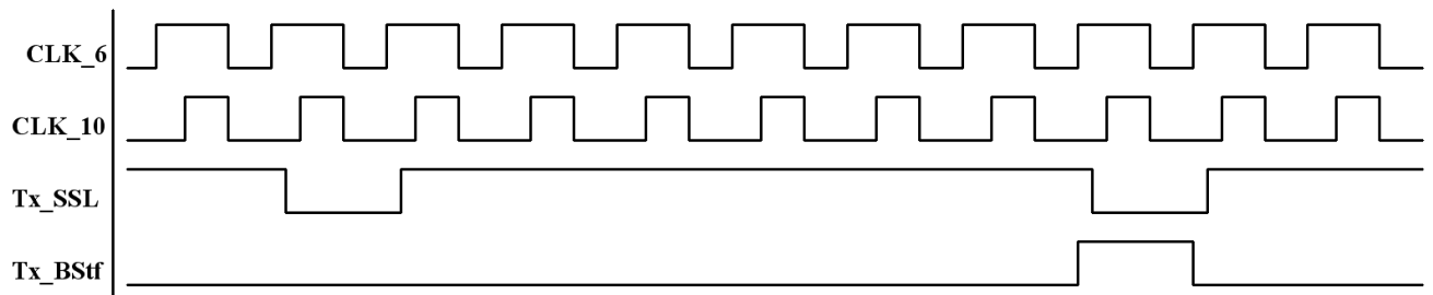
Rysunek 27: Działanie bloku wstawiania Bit Stuffing'u
