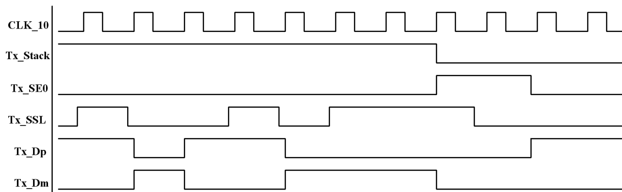
Rysunek 33: Działanie bloku konwertera zwykłego sygnału logicznego na NRZI
