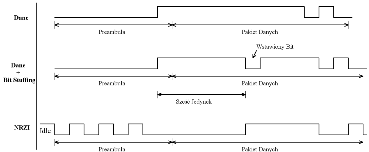
Rysunek 4: Zasada wstawiania bitów synchronizacyjnych
