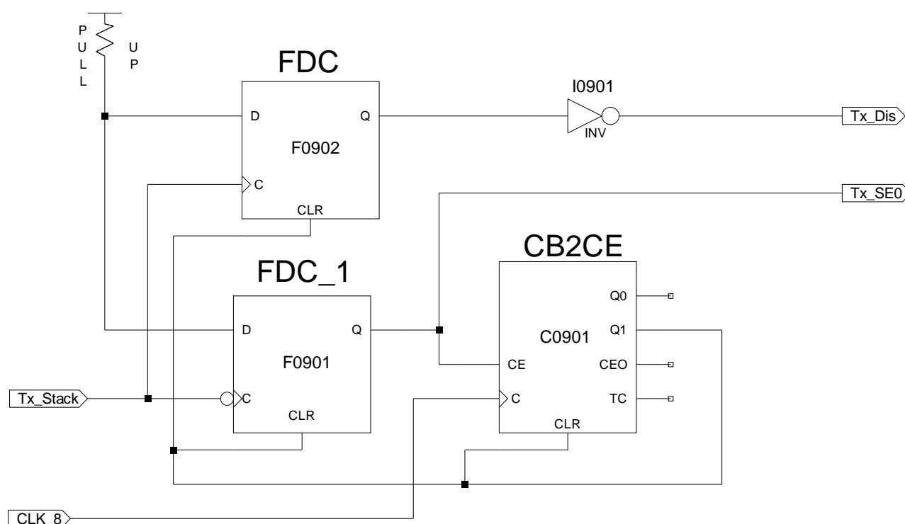
Rysunek 30: Schemat ideowy bloku generacji sygnału końca transmisji
