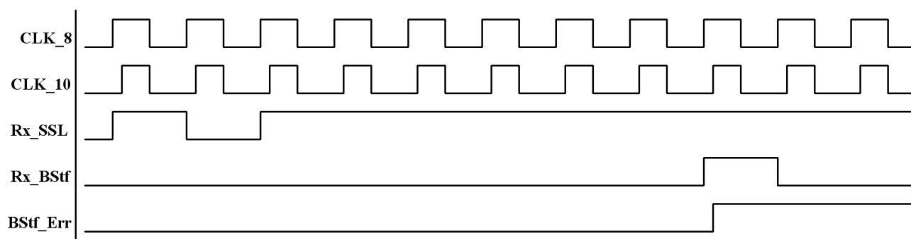
Rysunek 20: Sposób wykrywania błędów Bit Stuffing'u
