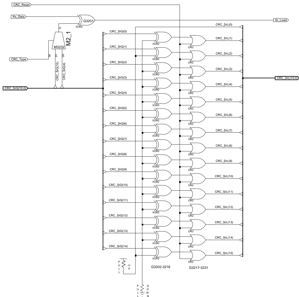
Rysunek 37: Dzielenie przez wielomian generacyjny CRC - schemat ideowy ( CRC_Div ).
