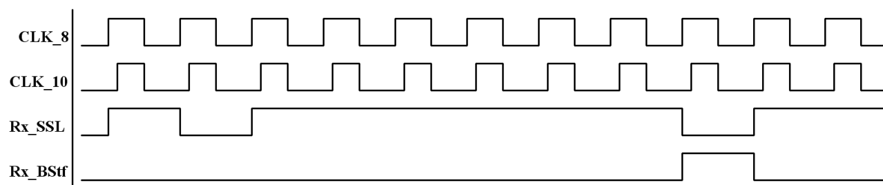
Rysunek 19: Działanie bloku wycinania Bit Stuffing'u
