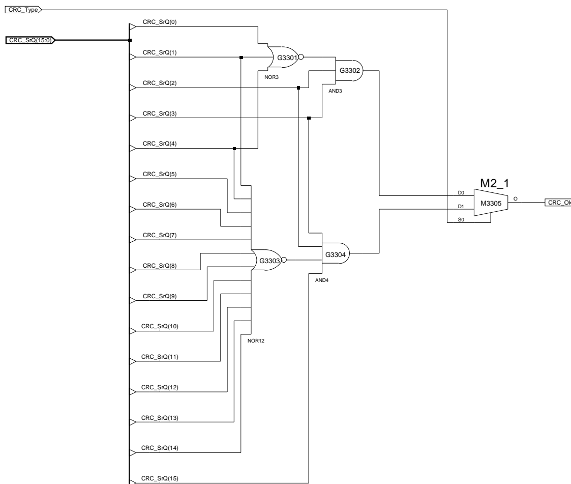
Rysunek 38: Kontrola poprawności reszty sumy kontrolnej - schemat ideowy ( CRC_Chk ).
