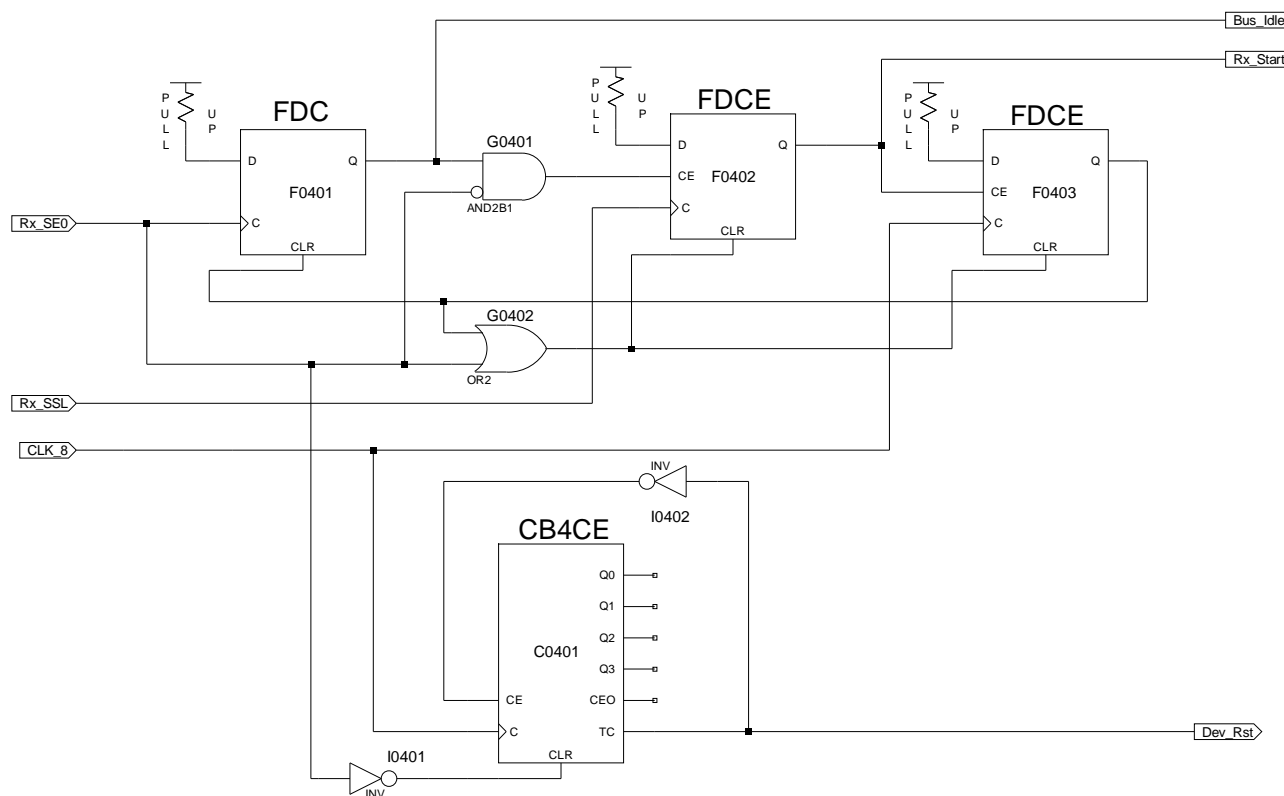
Rysunek 21: Schemat ideowy bloku monitorowania stanu transmisji
