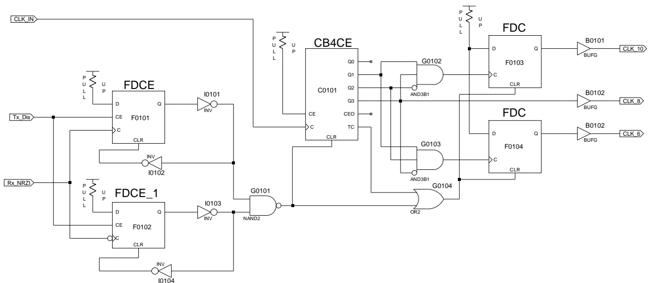
Rysunek 13: Schemat ideowy bloku odzyskiwania przebiegu zegarowego
