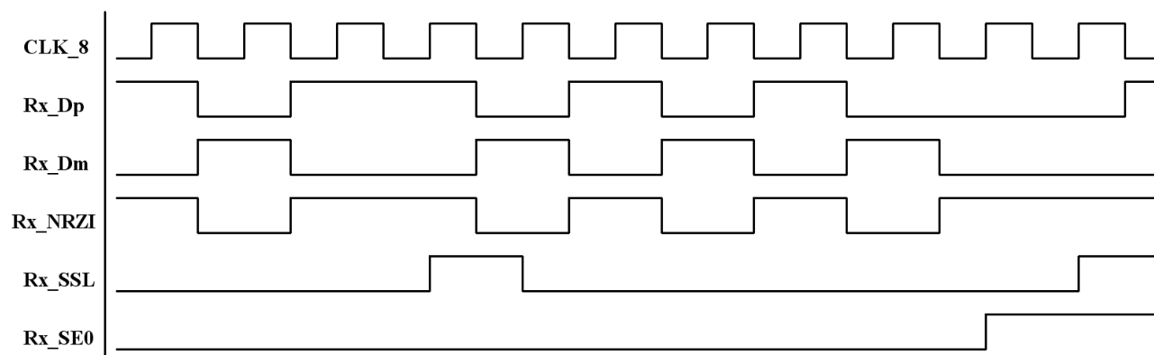
Rysunek 17: Wygląd przebiegów czasowych konwertera
