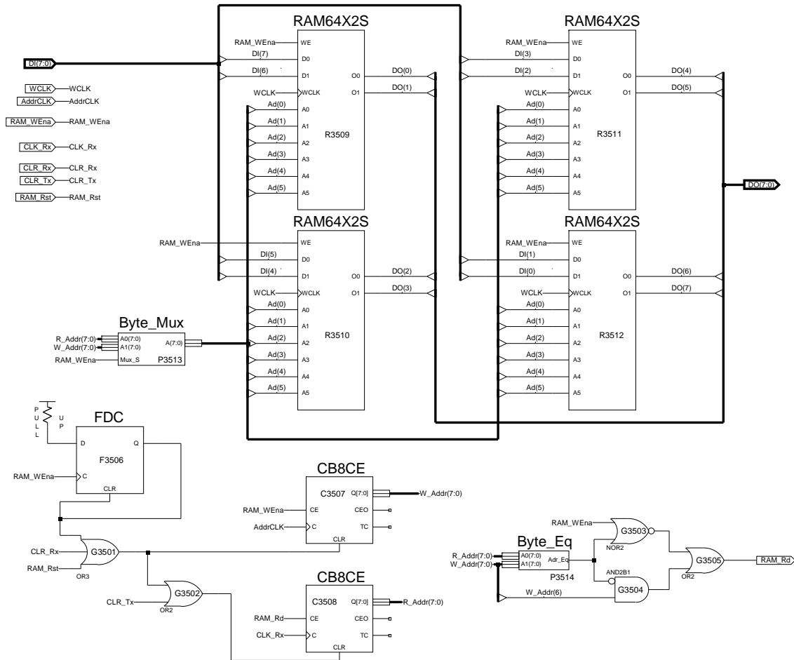
Rysunek 41: Pamięć RAM 64B - schemat ideowy (St_RAM64).
