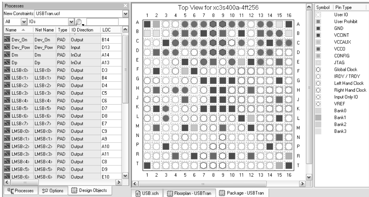
Rysunek 10: Ustawienia wyprowadzeń układu FPGA
